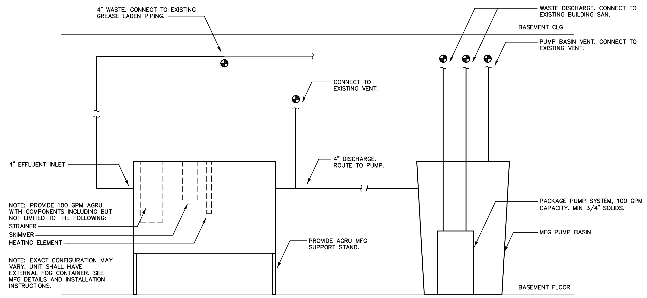
GREASE INTERCEPTOR/PUMP SCHEMATIC SCALE: N.T.S.
