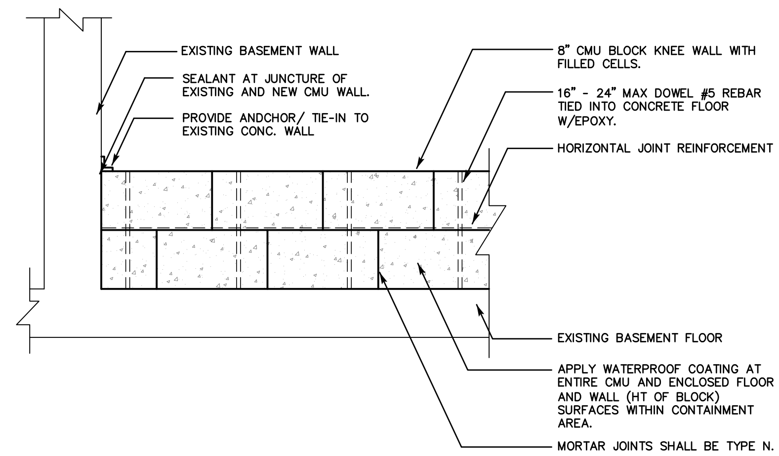
CMU CONTAINMENT AREA DETAIL SCALE: N.T.S.
